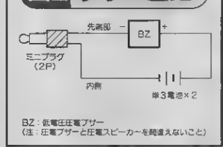
図2 ブザー回路
